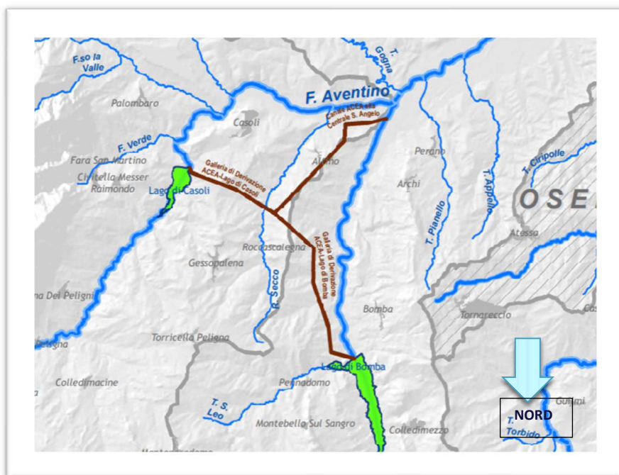
Figura 5: Layout geografico Impianto S. Angelo (estratto PTA Abruzzo Cartografia di Piano)_ Provincia di Chieti
