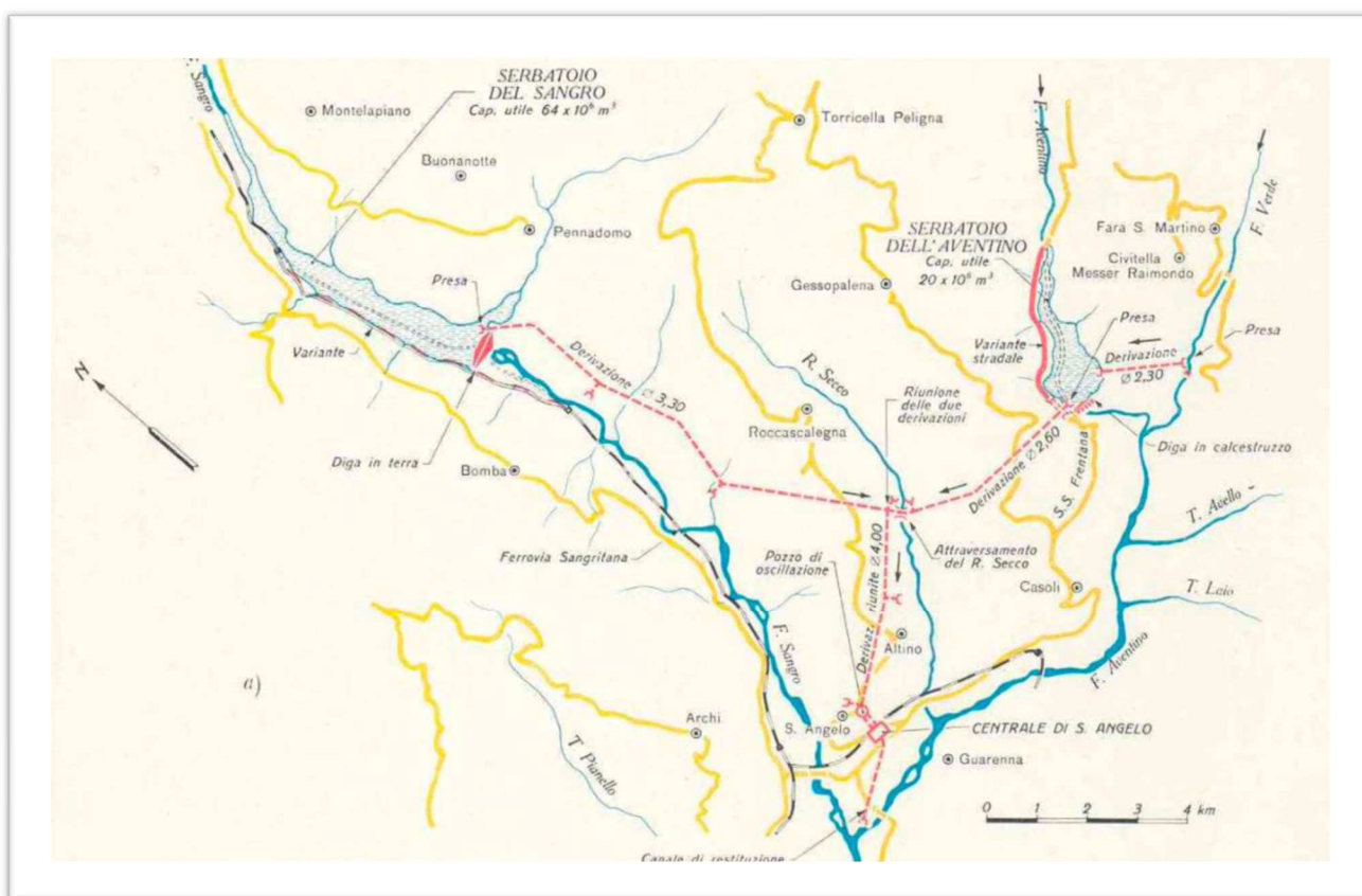
Figura 4: Dettaglio planimetrico dell'impianto idroelettrico "Sant'Angelo"
