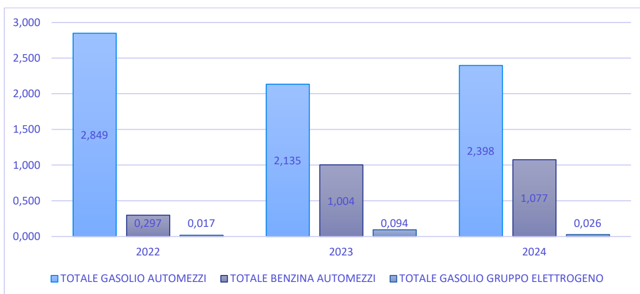
Figura 8: Consumi totali di Combustibili in TEP
